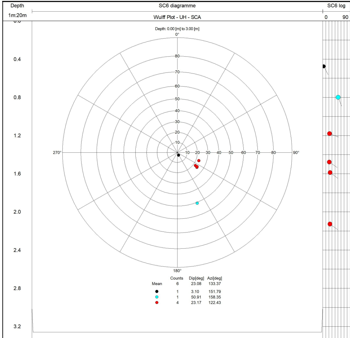
Figure 6 : Rose du sondage SC6
