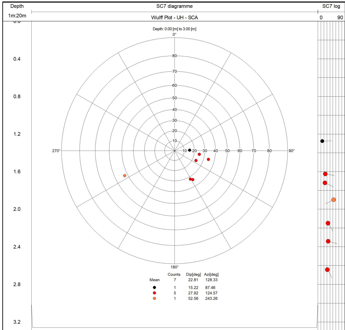
Figure 7 : Rose du sondage SC7
